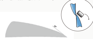
【コンベックス刃断面図(38度)】
