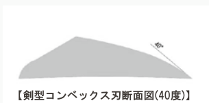
【剣型コンベックス刃断面図(40度)】
