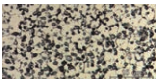
パウダーメタルアロイ：微細で均一な金属組織 一般的な刃物鋼：粗く、不揃いな金属組織
