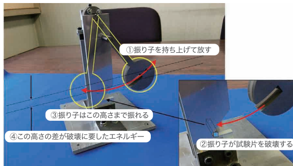
シャルピー衝撃試験機
